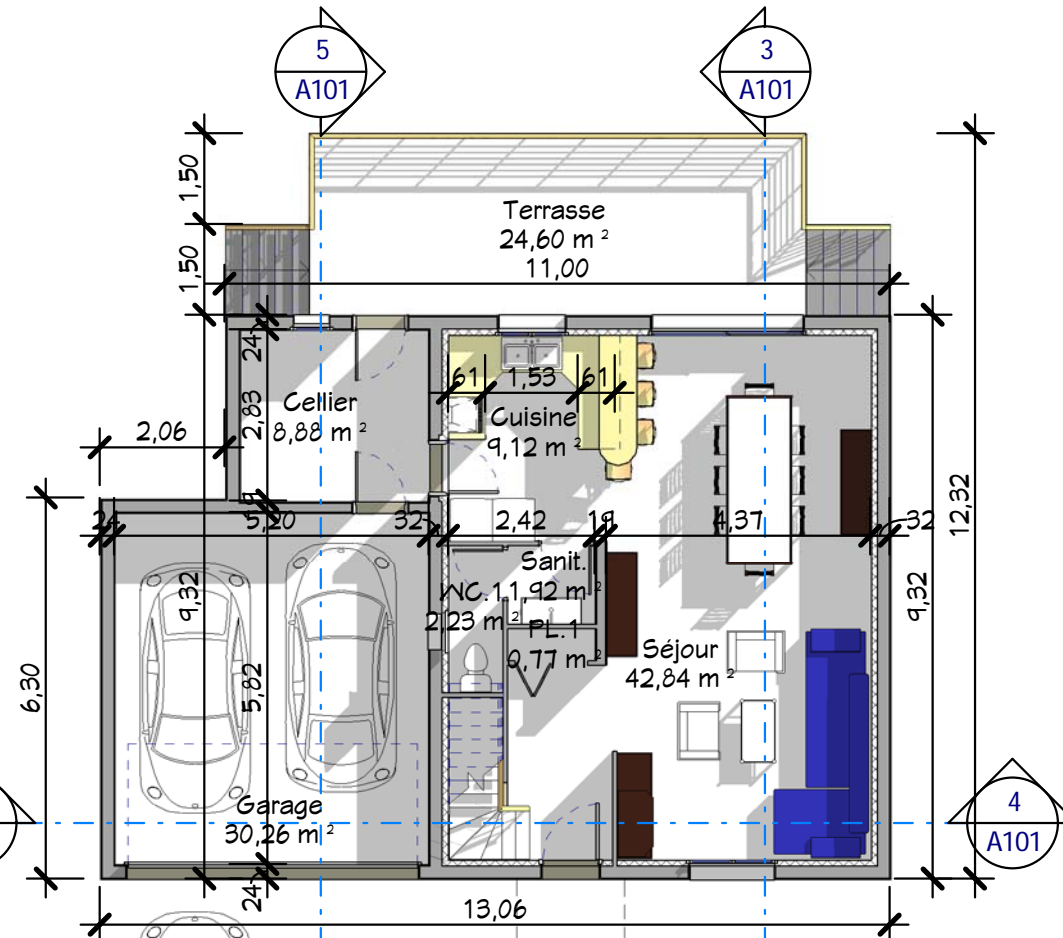
1 RDC Ech : 1 : 125
