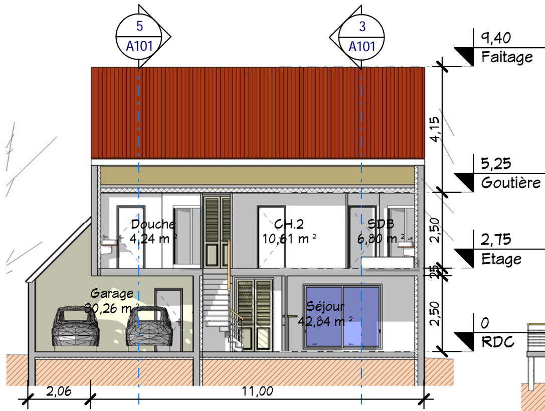
4 Coupe 2 Ech : 1 : 125
