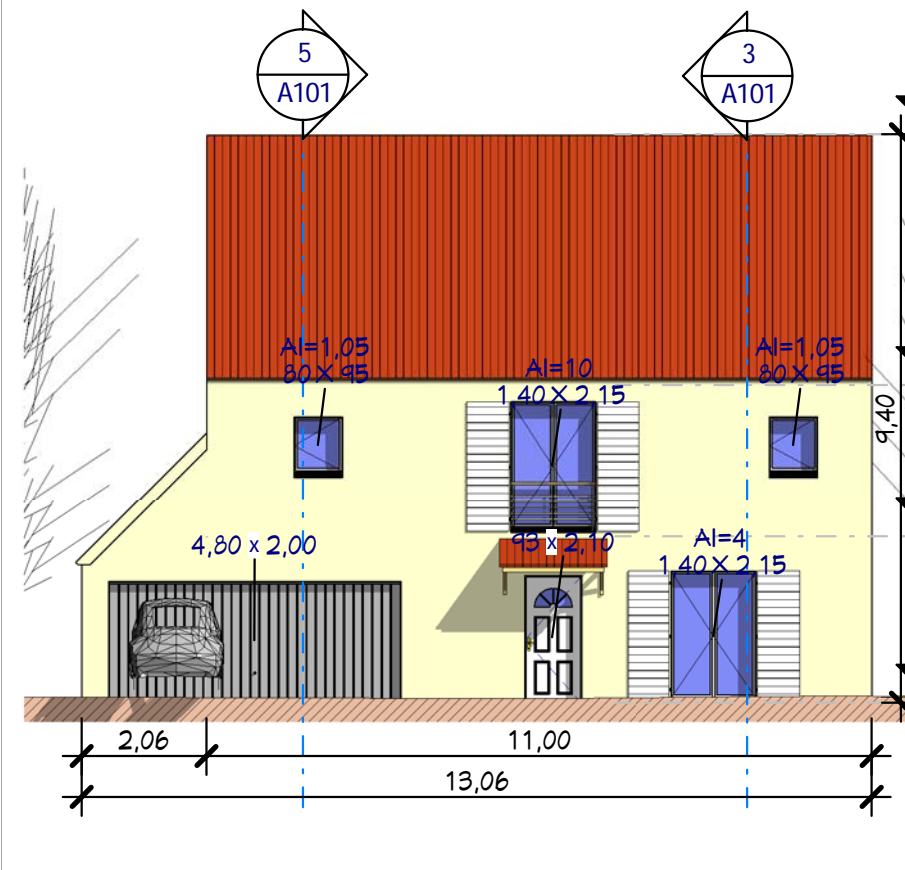
2 Elév. Est Ech : 1 : 125
