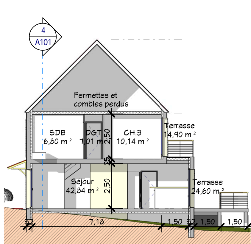
3 Coupe 1 Ech : 1 : 125
