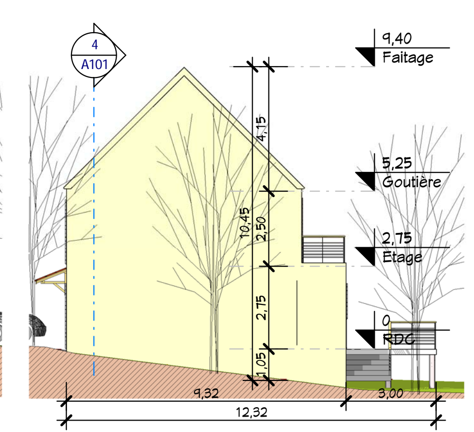
5 Elév. Nord Ech : 1 : 125
