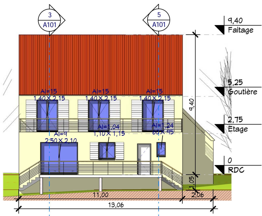
3 Elév. Ouest Ech : 1 : 125
