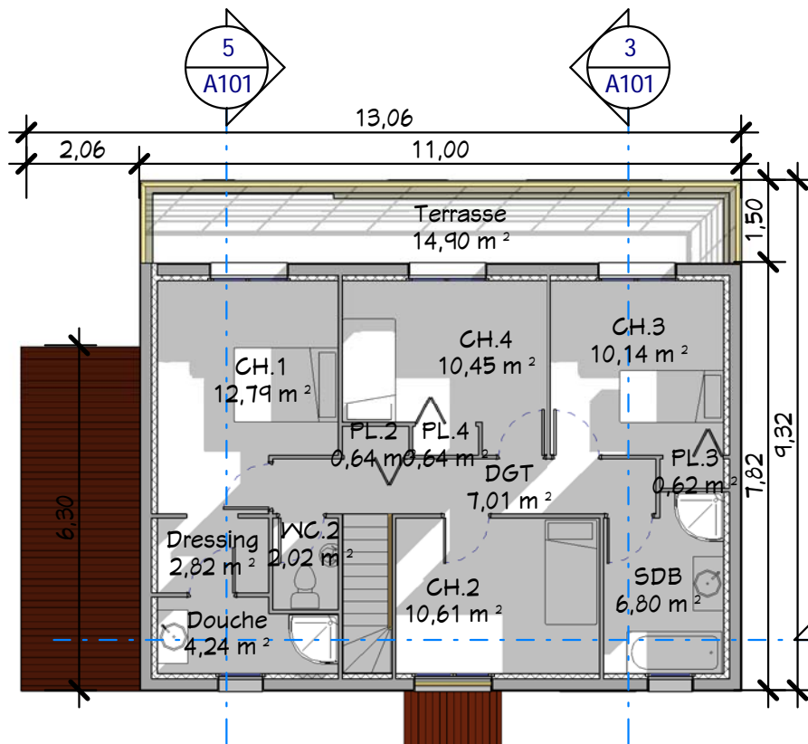
2 Etage Ech : 1 : 125
