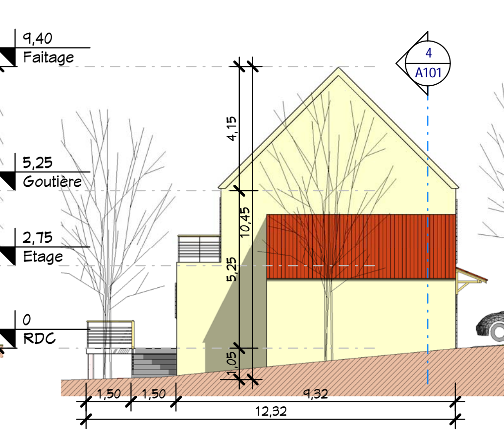
4 Elév. Sud Ech : 1 : 125
