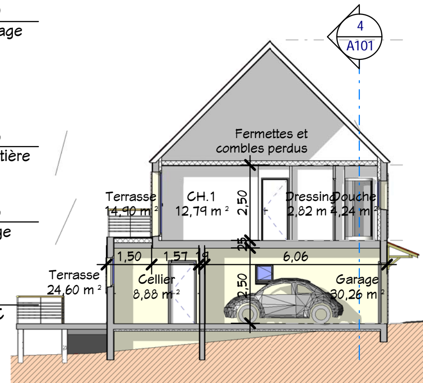
5 Coupe 3 Ech : 1 : 125
